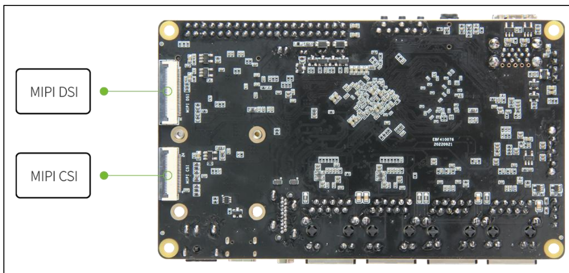
图 3.2.1-3 鲁班猫 2N 背面视图
