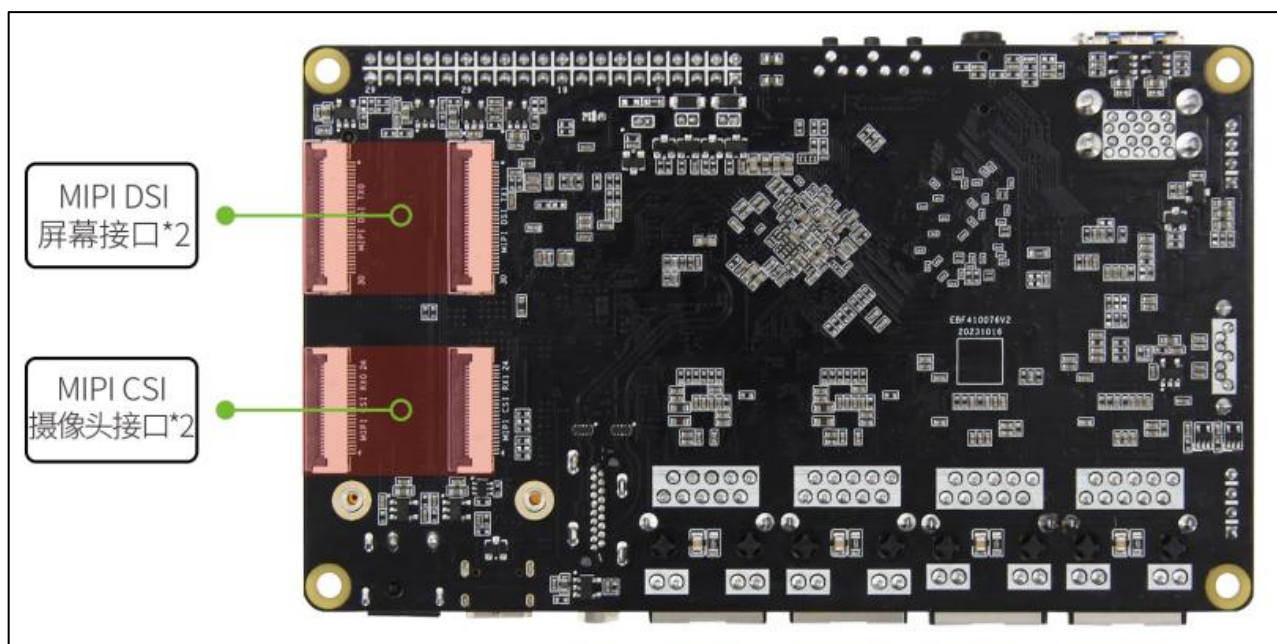
图 3.2.1-6 鲁班猫 2N-V2 背面视图
