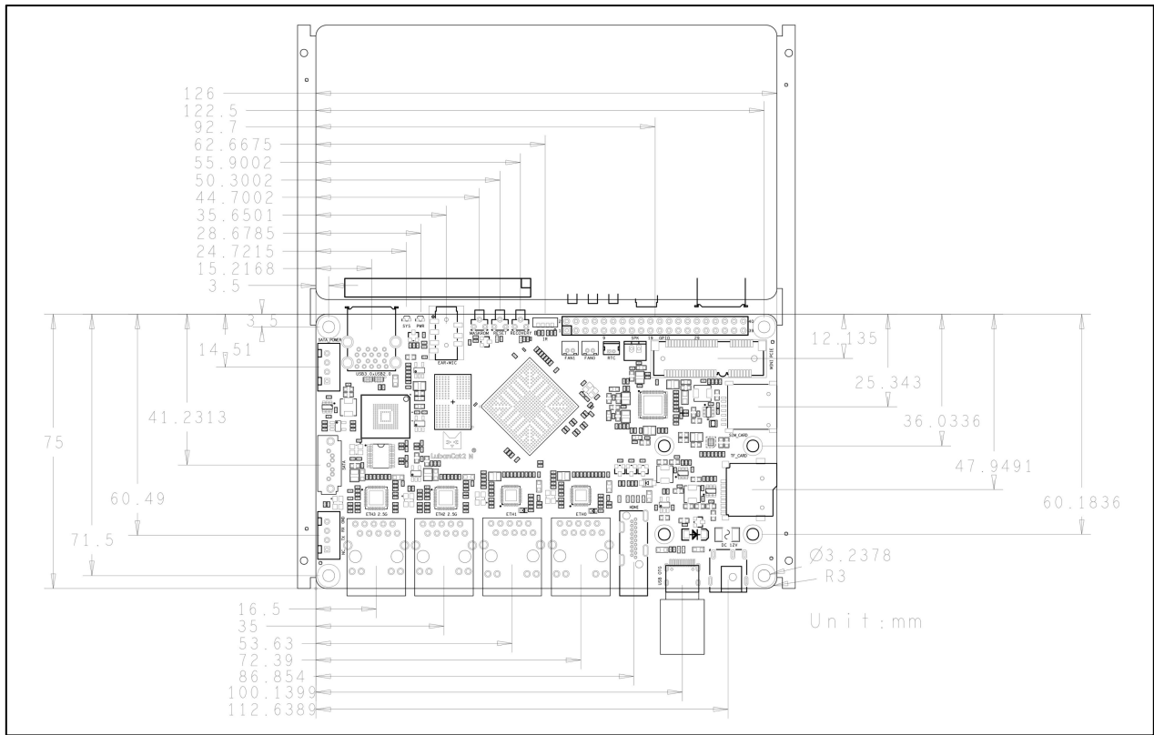
图 3.2.2-1 鲁班猫 2N 机械尺寸图
