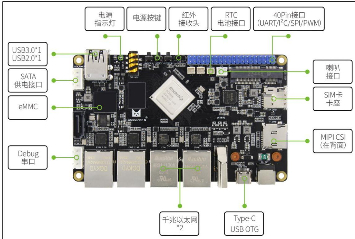
图 3.2.1-1 鲁班猫 2N 正面标注视图 1
