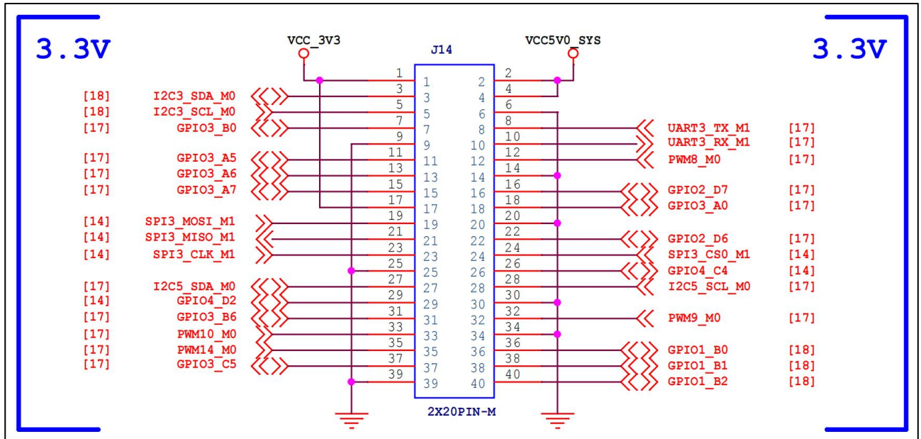
图 3.6-1 鲁班猫 2N 引脚原理图
