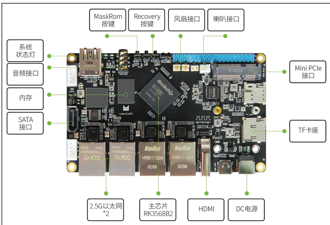
图 3.2.1-5 鲁班猫 2N-V2 正面标注视图 2
