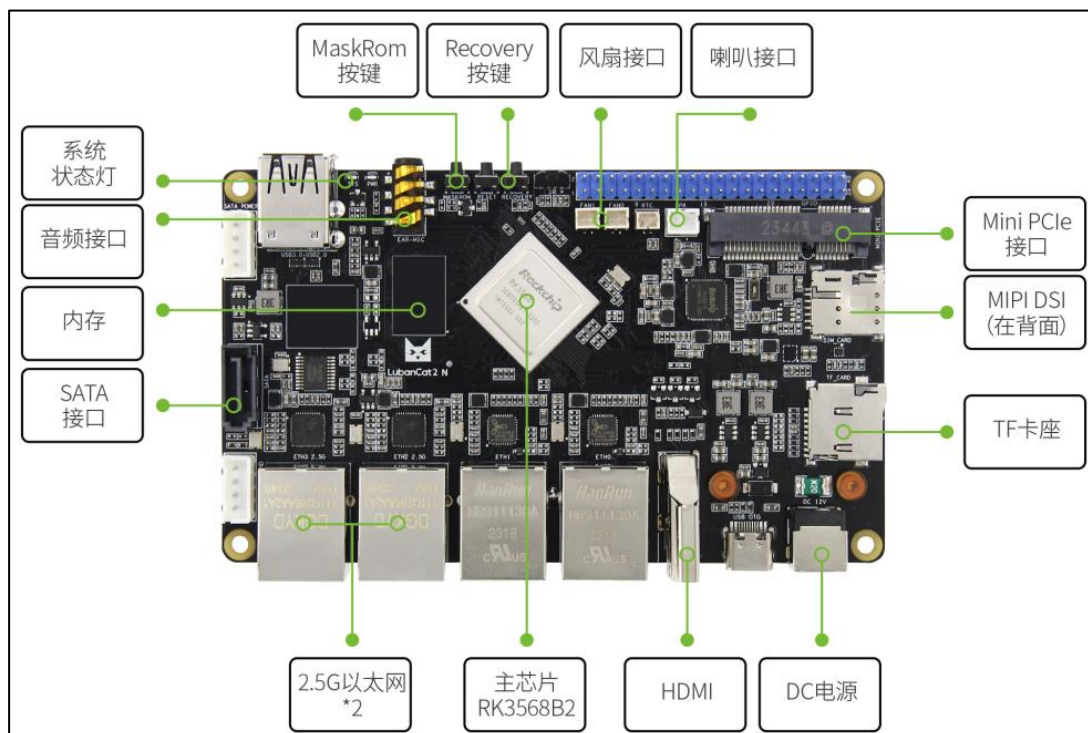
图 3.2.1-2 鲁班猫 2N 正面标注视图 2
