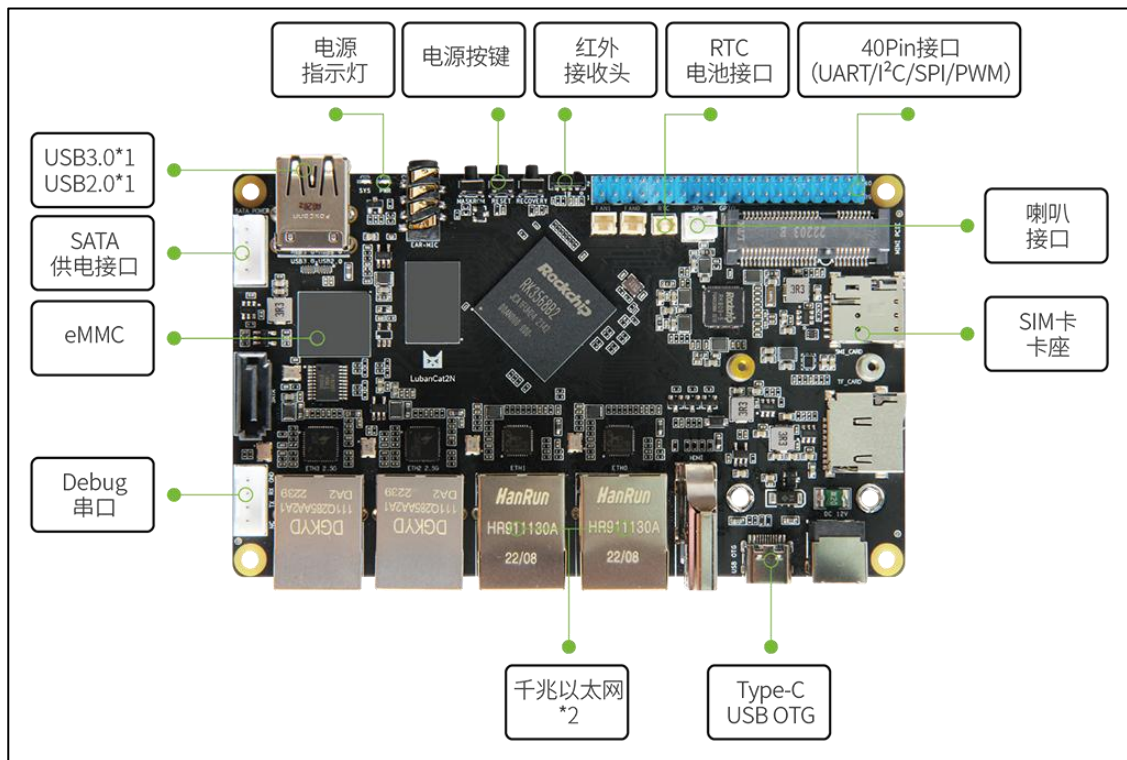
图 3.2.1-4 鲁班猫 2N-V2 正面标注视图 1
